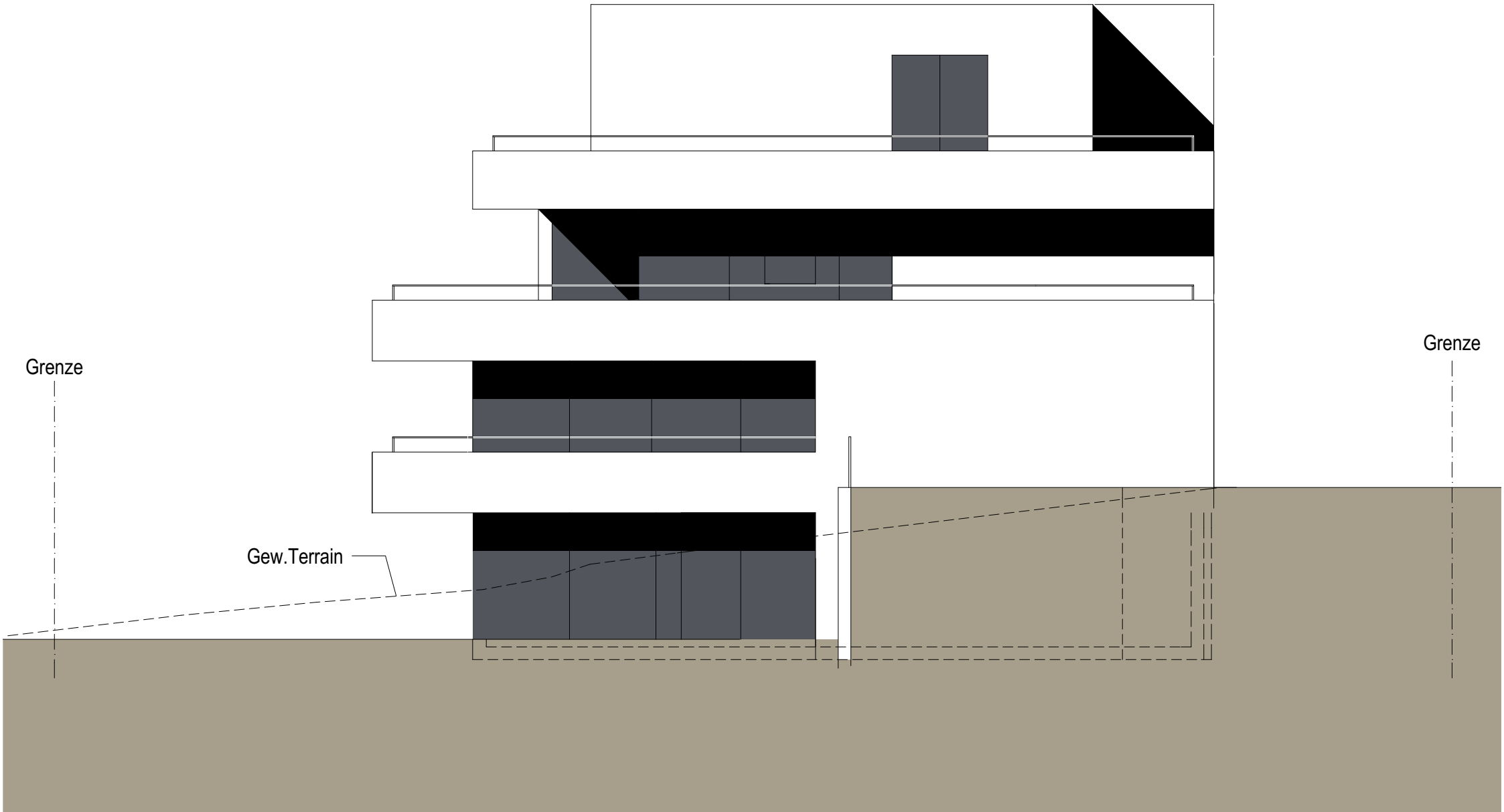
Ansicht Ost
